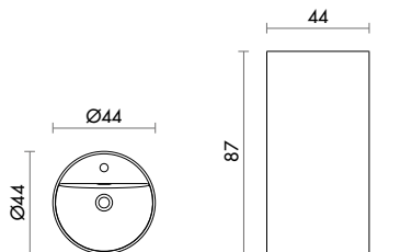
DIM. VASCA L.42 P.29,4 H.12,4 TANK DIMENSIONS L.42 P.29,4 H.12,4
